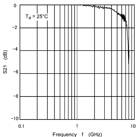
Fig. 10.1 S_{21} - f
