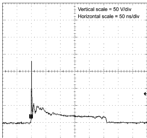
Fig. 11.1 +8 kV
