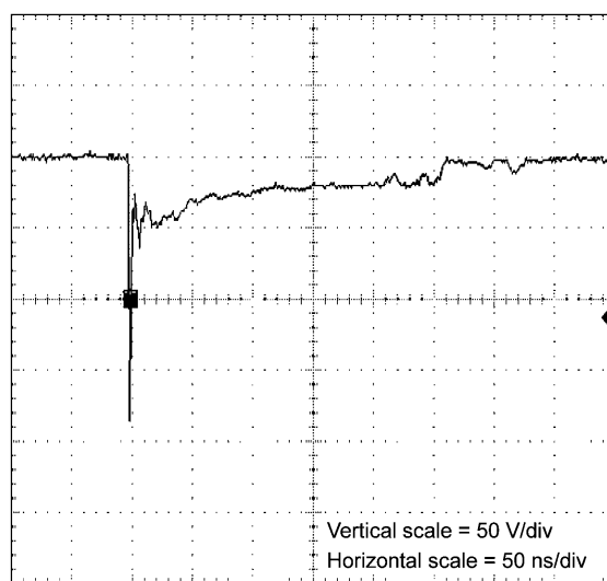
Fig. 11.2 -8 kV
