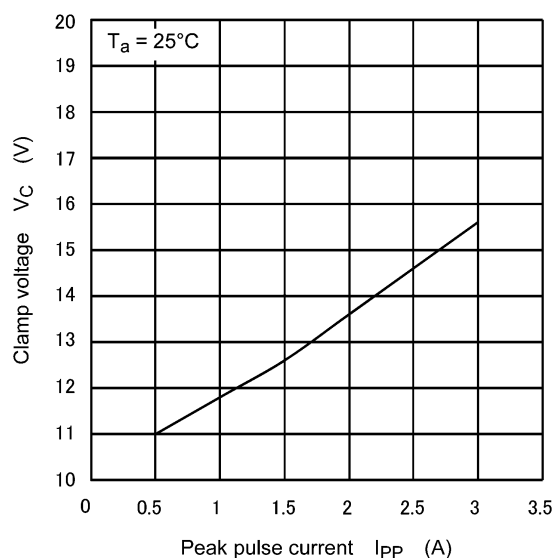
Fig. 9.1 V_C - I_{PP}
