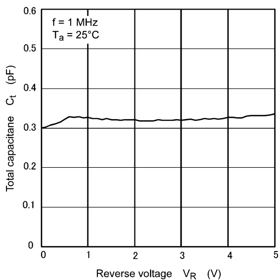
Fig. 8.3 C_t - V_R
