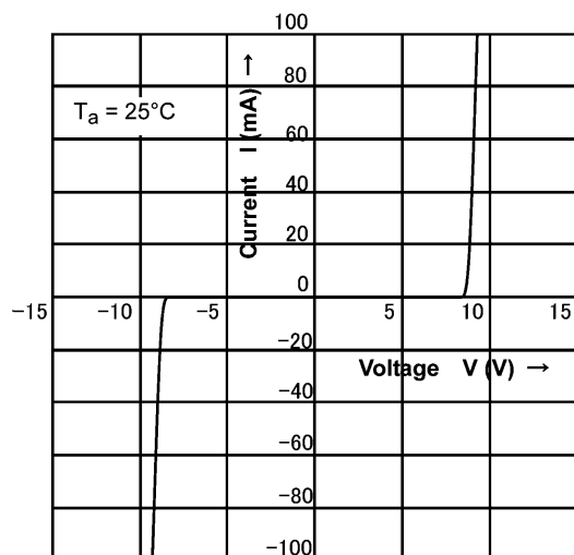
Fig. 8.1 I - V
