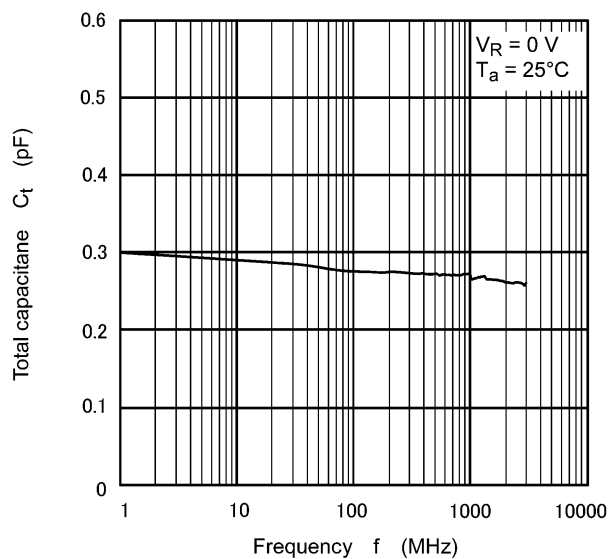
Fig. 8.4 C_t - f
