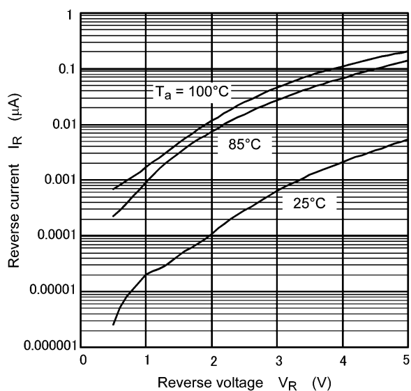
Fig. 8.2 I_R - V_R
