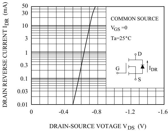
I_{DR} - V_{DS}
