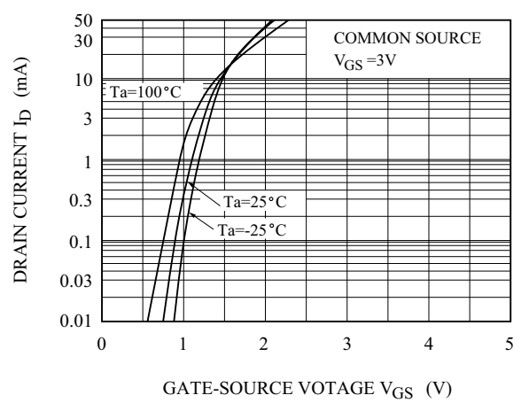
I_D - V_{GS}
