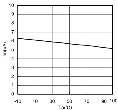
Fig.34 Ta-Ien
