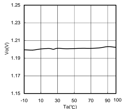
Fig.27 Ta-Vo (Io=0mA)
