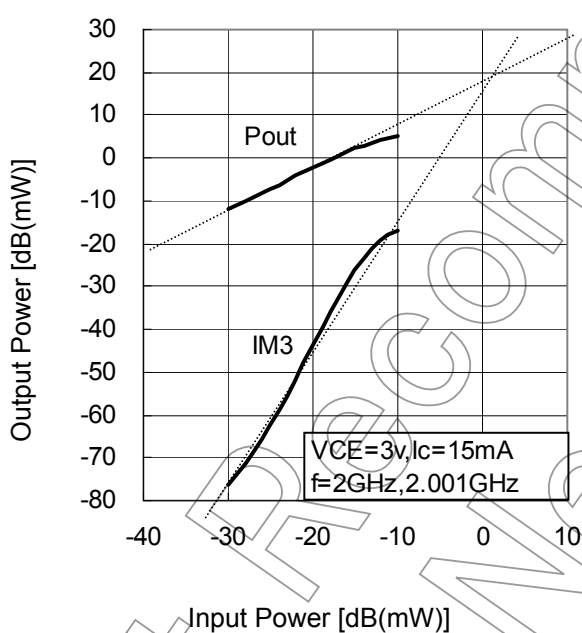
IM3 (2GHz)
