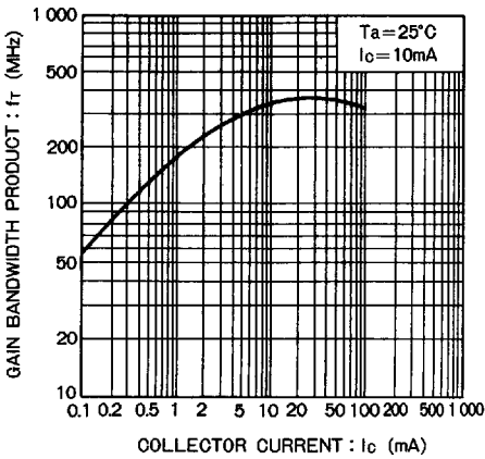
Fig. 7 利得帯域幅積-コレクタ電流特性
