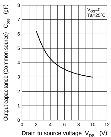
C_{oss} - V_{DS}
