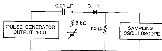
逆回復時間 (trr) 測定回路
