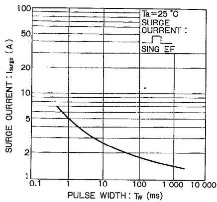
Fig.5 サージ電流特性
