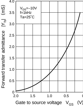
|Y_{fs}| - V_{GS}
