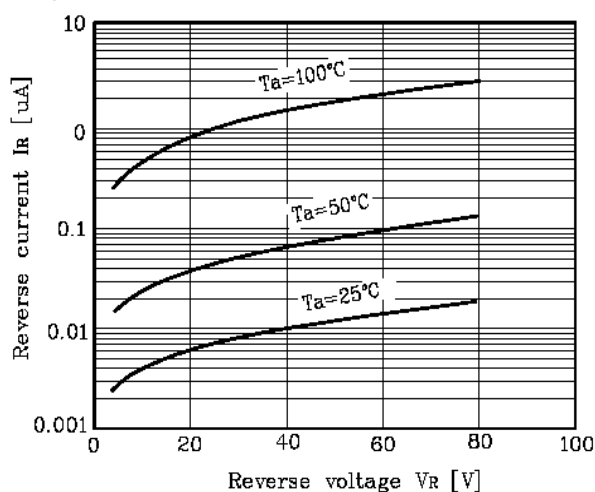
Fig 2. I_R - V_R
