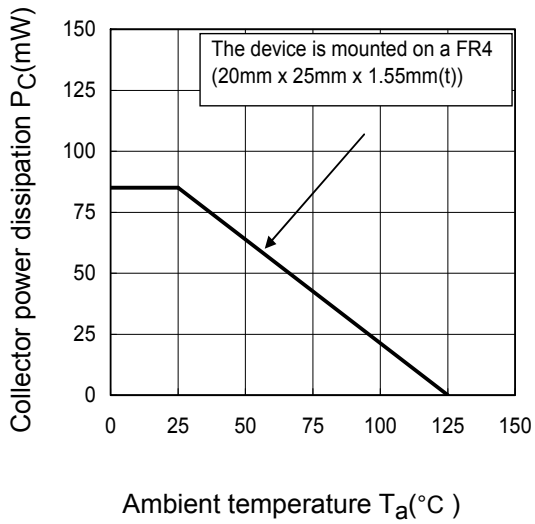
P_C - T_a
