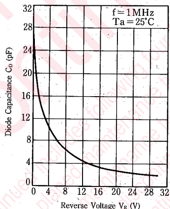
C_D - V_R
